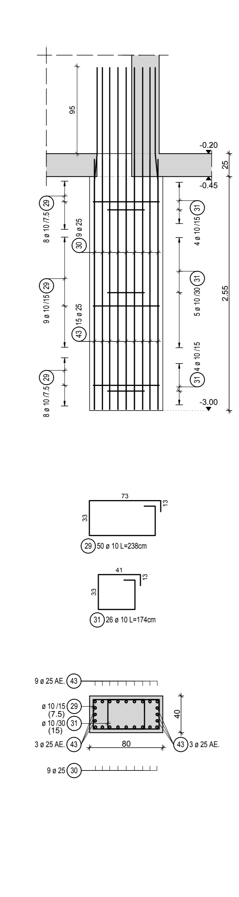
2x Stb. Stütze b/h=80/40cm (C35/45, XD3, XF1, WF) Pos. S56, Pos. S57
