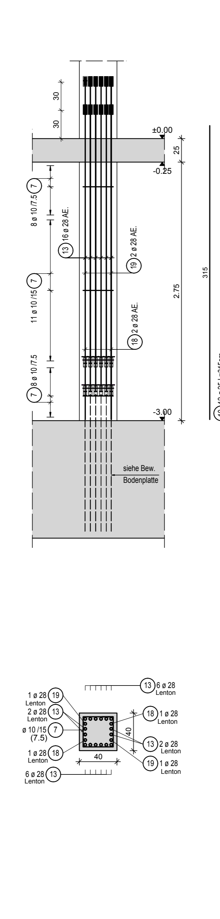
Stb. Stütze b/h=40/40cm (C35/45, XD3, XF1, WF) Pos. S23
