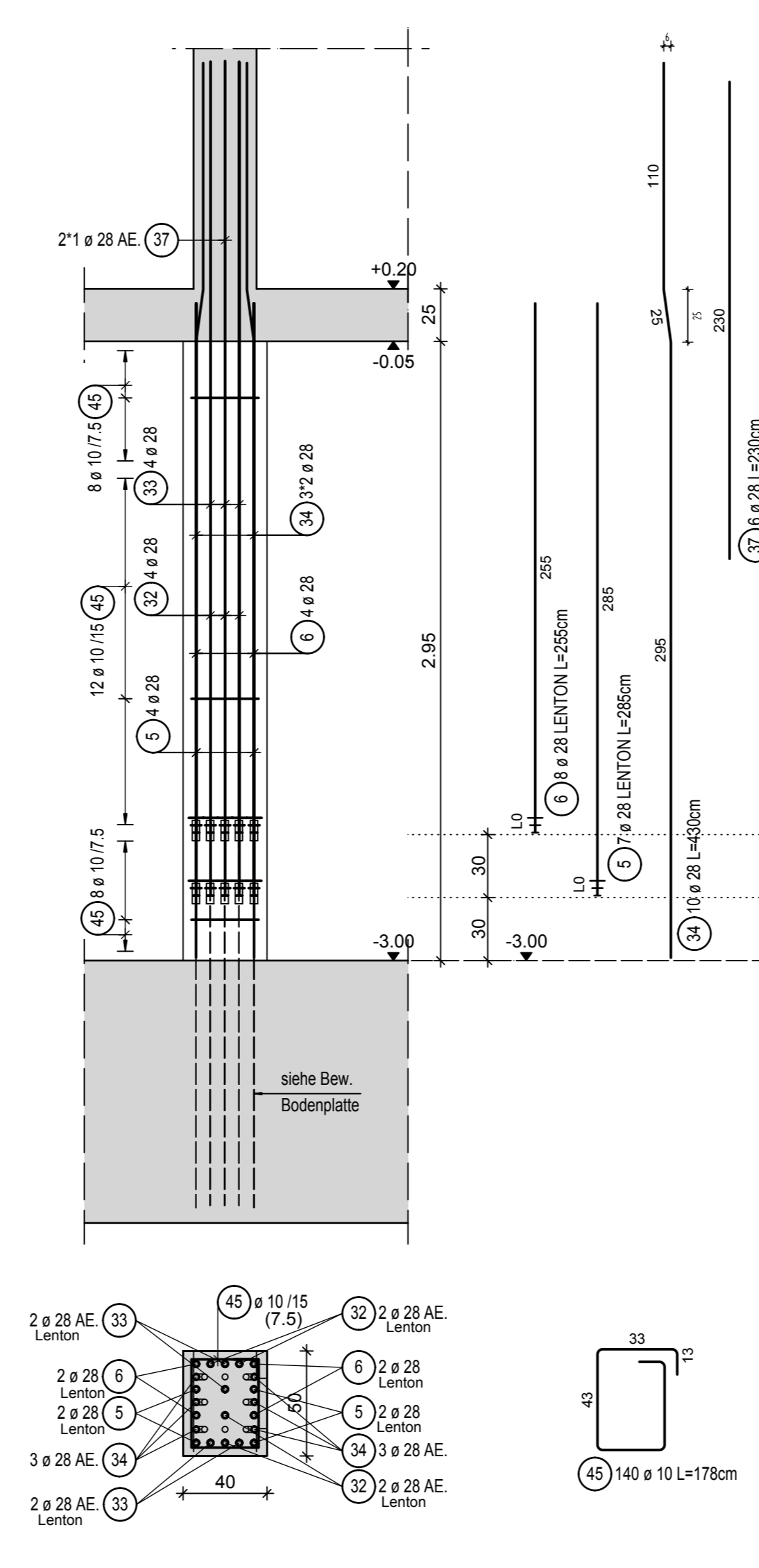
Stb. Stütze b/h=40/50cm (C35/45, XD3, XF1, WF) Pos. S50
