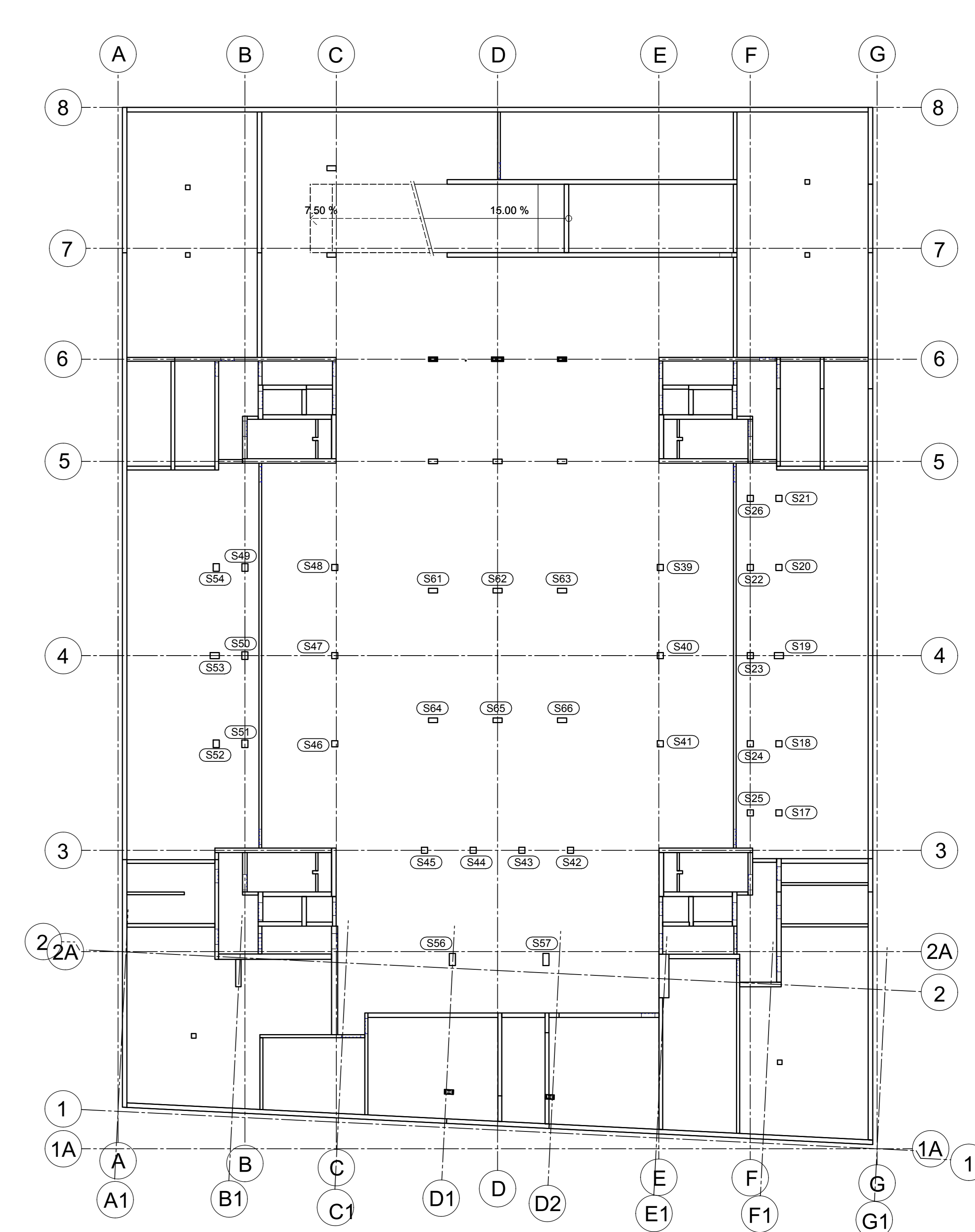
Übersicht M.1:200
