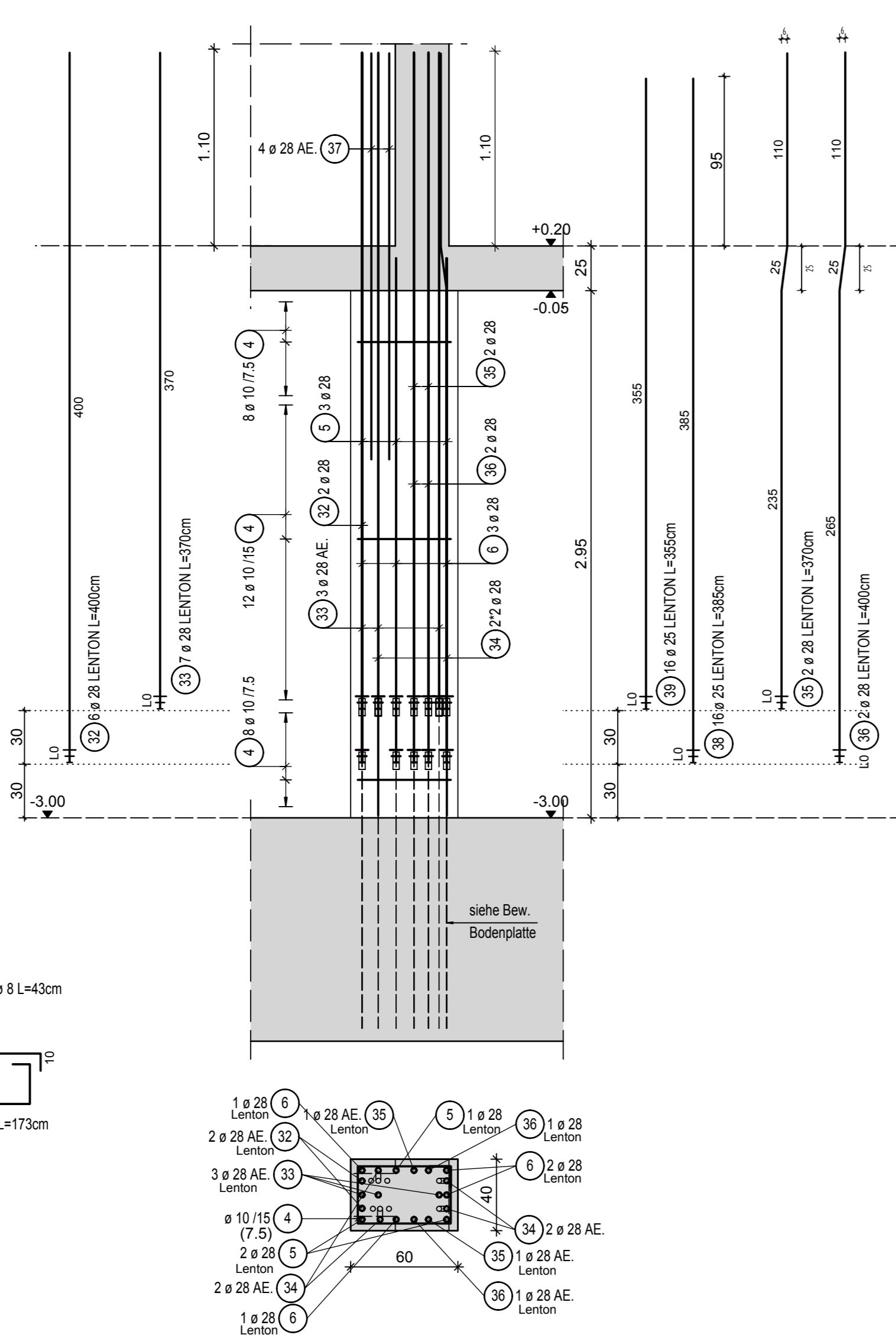
Stb. Stütze b/h=60/40cm (C35/45, XD3, XF1, WF) Pos. S53
